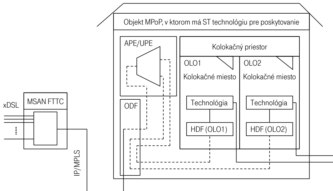
Obr. 3 – Fyzická kolokácia v prípade technológie xDSL FTTC
