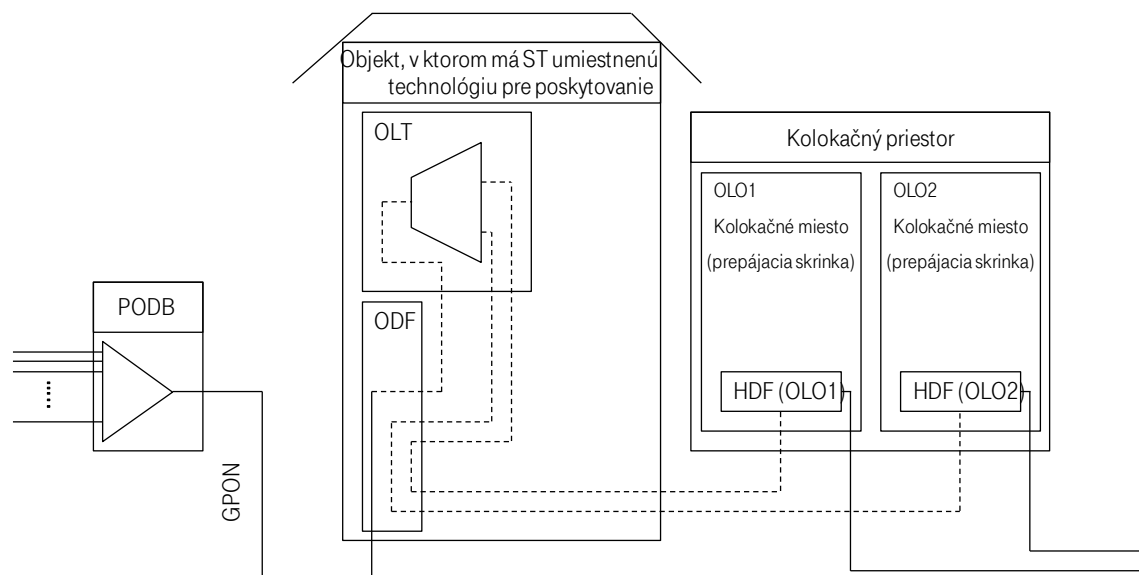
Obr. 2 – Vzdialená kolokácia v prípade technológie GPON FTTH
