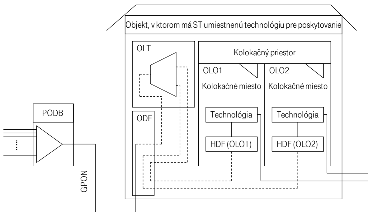
Obr. 1 – Fyzická kolokácia v prípade technológie GPON FTTH
