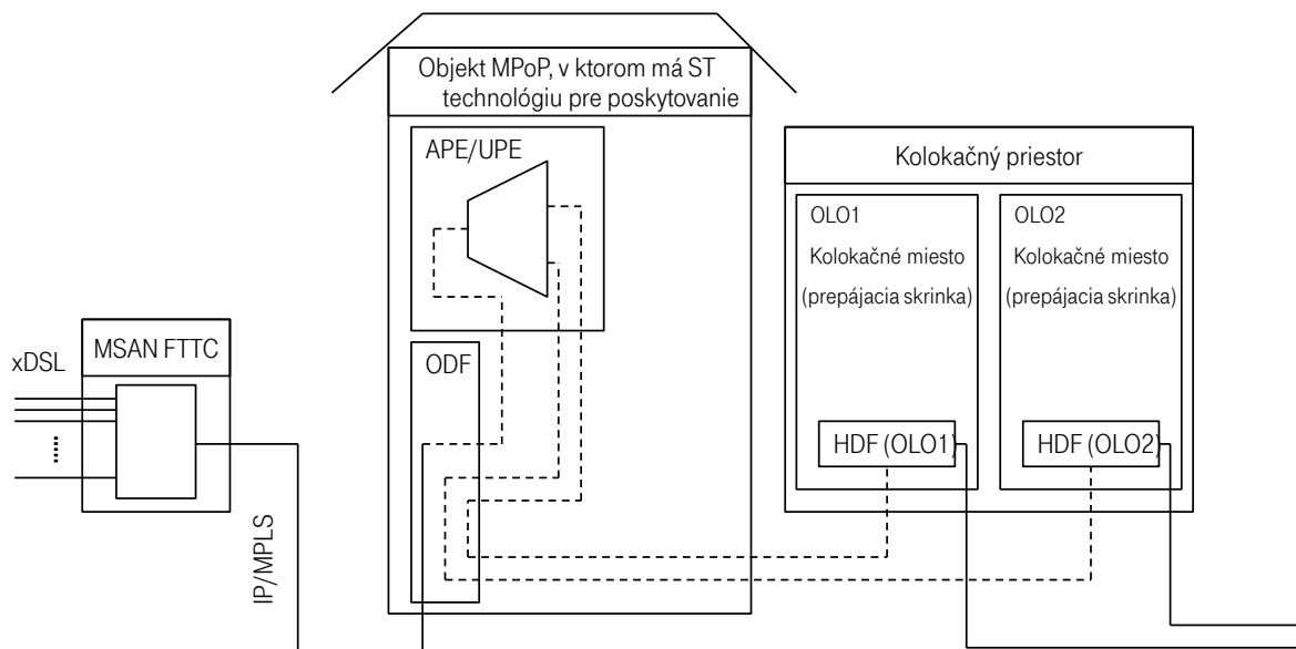
Obr. 4 – Vzdialená kolokácia v prípade technológie xDSL FTTC
